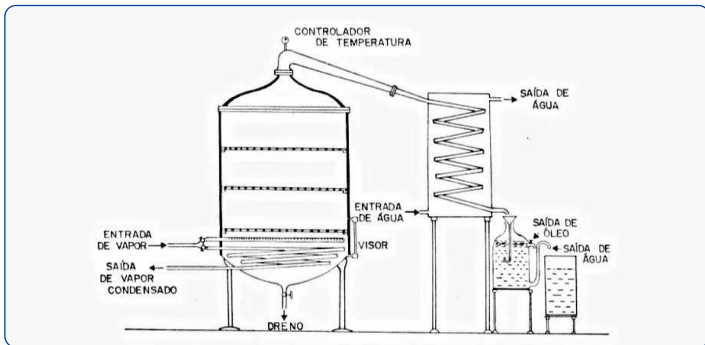
Figura 2: Hidrodestilação.
