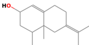
Figura 9: \alpha -Vetivol.
